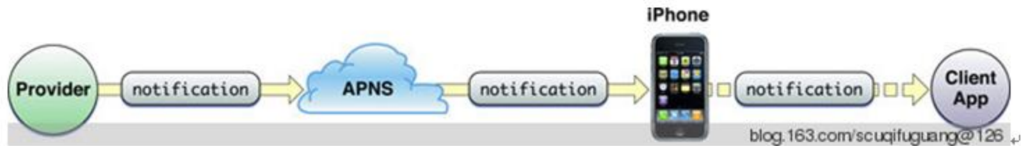
图 1 APNS 推送流程
